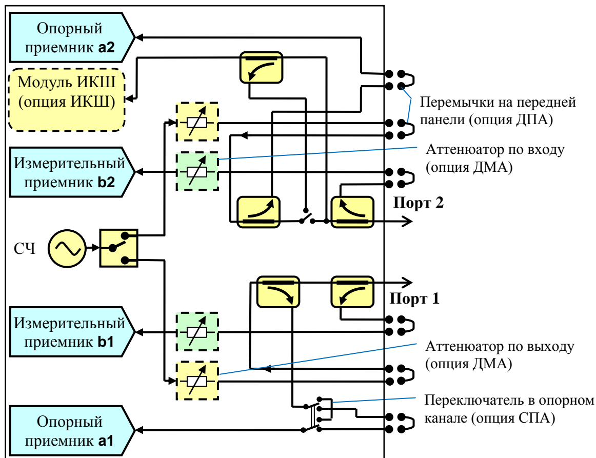
Рисунок 4.1 – Структурная схема
