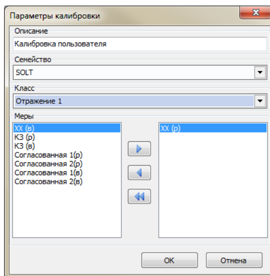
Рисунок Б.8 – Окно параметров калибровки
