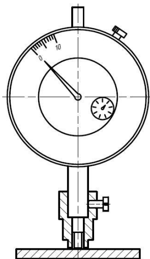
Рисунок 3.2 – Установка нуля
