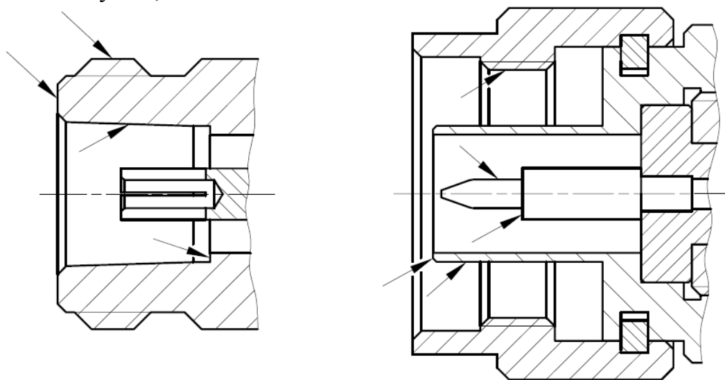
Рисунок 3.1 – Очищаемые поверхности
