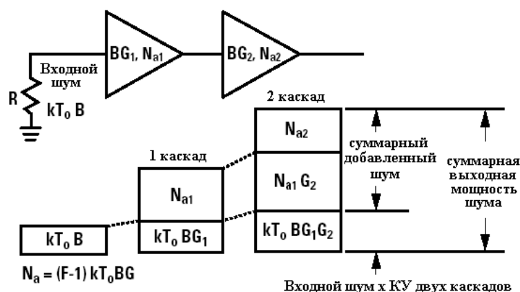
Рисунок 4.9 – Иллюстрация влияния второго каскада на измерение КШ
