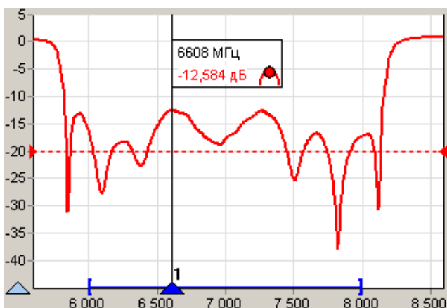
Рисунок 3.27 – Следящий маркер
