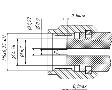
Соединитель тип IX, вар. 1 (вилка)
