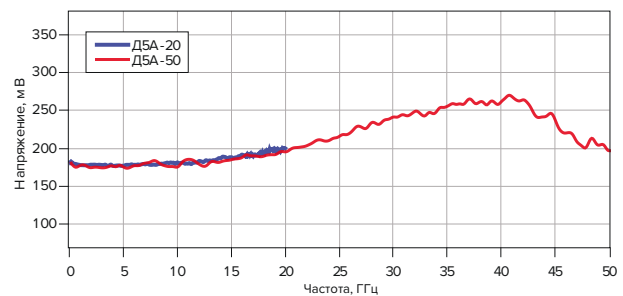
Частотная характеристика (при входной мощности 0 дБм)
