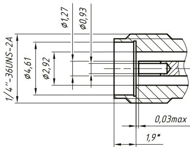
Соединитель тип 2,92 мм (розетка)
