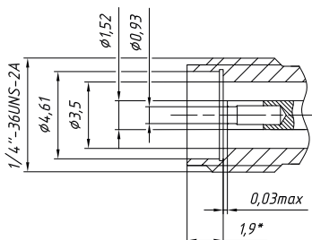
Соединитель тип 3,5 мм (розетка)
