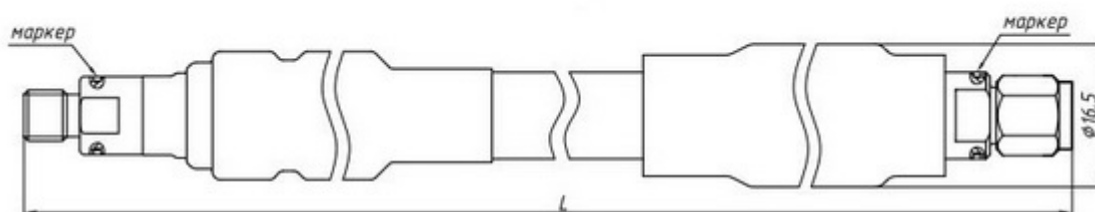
Кабельная сборка КСА20А-13Р-03
