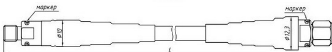
Кабельная сборка КС20А-13Р-03
